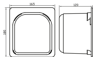
Gran Formato 2,5 l. 122 x 180 x 165 mm. (alto x largo x ancho)
