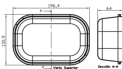
Tarrina 1 l. 64 x 196,4 x 130,9 mm. (alto x largo x ancho)
