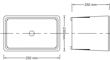
Gran Formato 8 l. 250 x 250 x 230 mm. (alto x largo x ancho)
